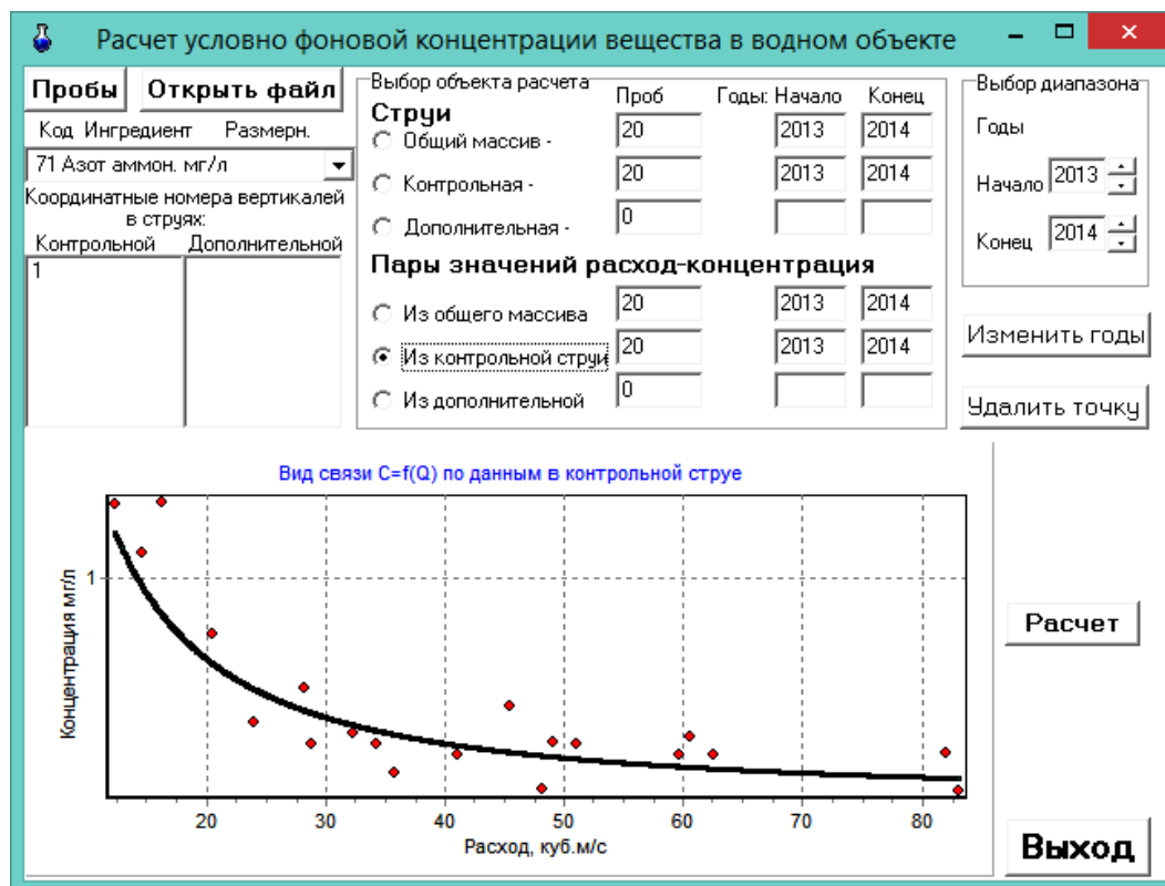
Рисунок Г.1 – Зависимость изменения концентрации азота аммонийного от расхода речной воды в створе N реки А
